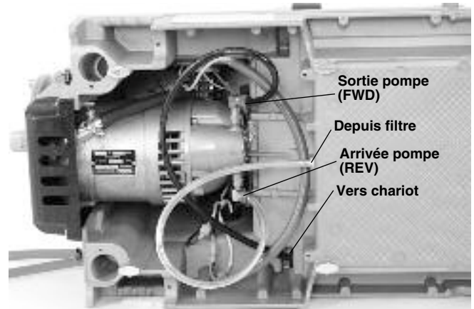
Figure 25B – Raccordement de pompe à huile pour filetages à droit (interrupteur en position FWD)
