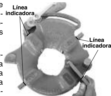
Figura 8 – Inserción de terrajas
