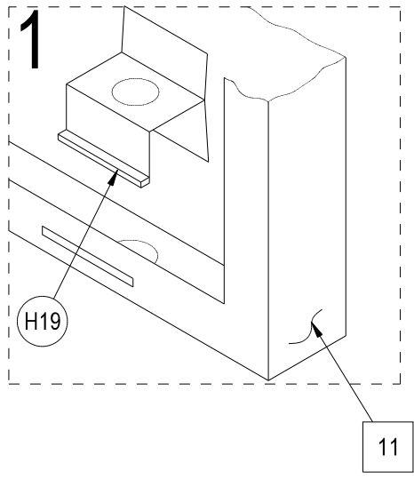
RIGHT DOOR ROD ASSEMBLY
